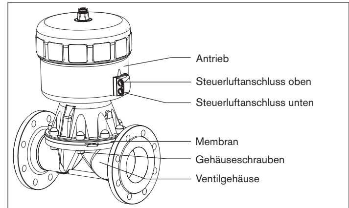
Bild 10: Montage
