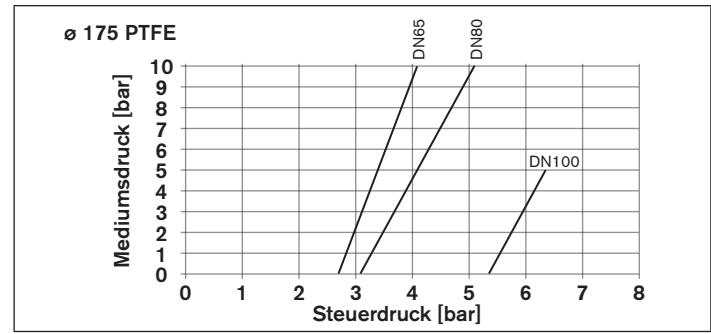
Bild 8: Druckdiagramm, Antrieb ø 175 mm, Steuerfunktion B, PTFE-Membran
