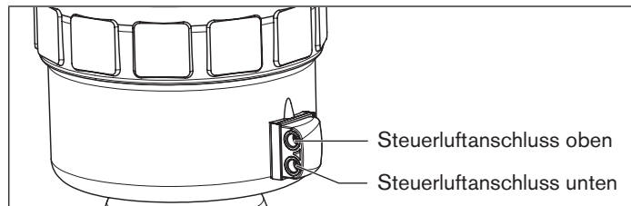
Bild 14: Pneumatischer Anschluss
