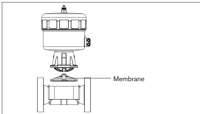
Fig. 16 : Pièce de rechange membrane
