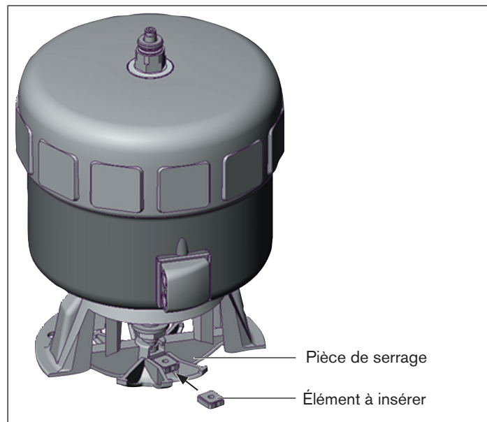
Fig. 13 : Montage d' l'élément à insérer
