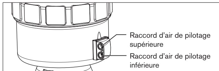
Fig. 12 : Raccord d'air de pilotage
