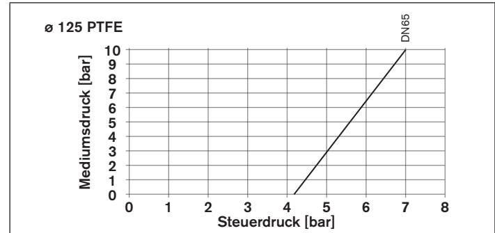
Bild 7: Druckdiagramm, Antrieb ø 125 mm, Steuerfunktion B, PTFE-Membran
