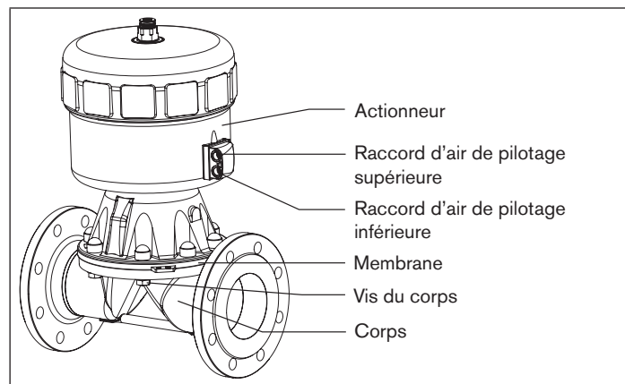
Fig. 10 : Montage
