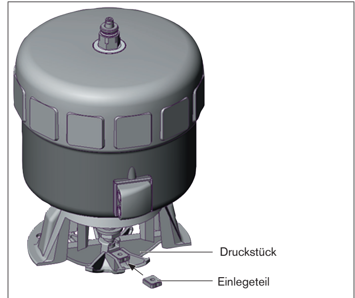
Bild 13: Montage Einlegeteil
