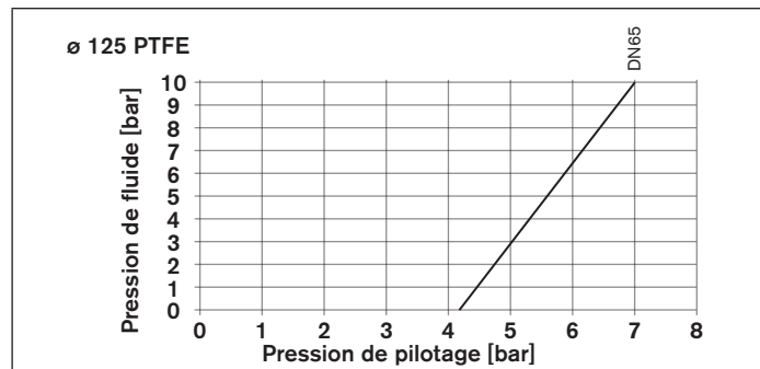
Fig. 8 : Diagramme de pression, actionneur ø 175 mm, fonction B, membrane PTFE
