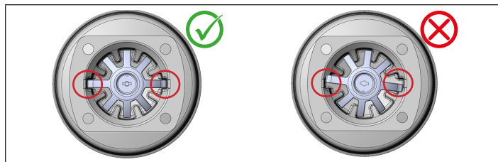
Fig. 11 : Position correcte et incorrecte de la pièce à presser
