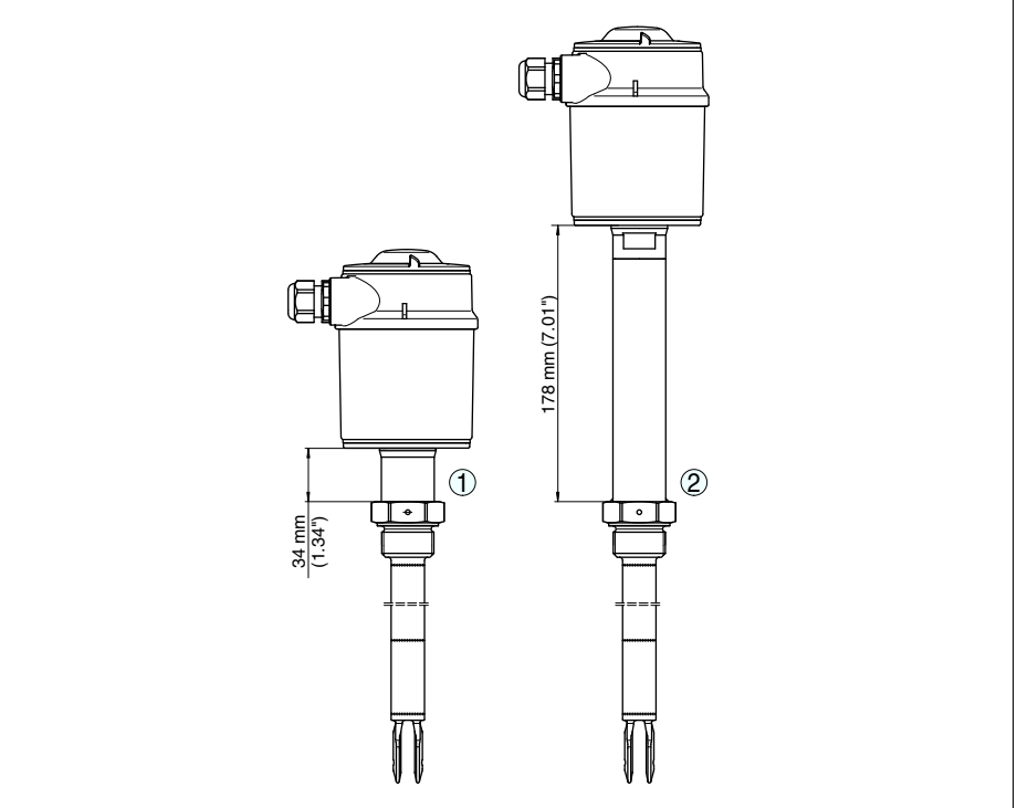
Fig. 37: Options
