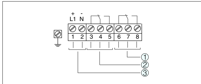
Fig. 11: Schéma de raccordement boîtier à chambre unique
