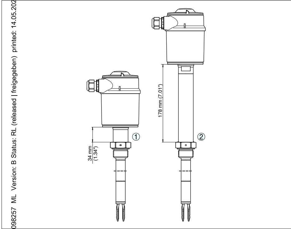
Abb. 34: Optionen
