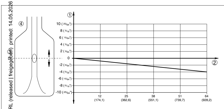
Abb. 28: Einfluss des Prozessdrucks auf den Schaltpunkt
