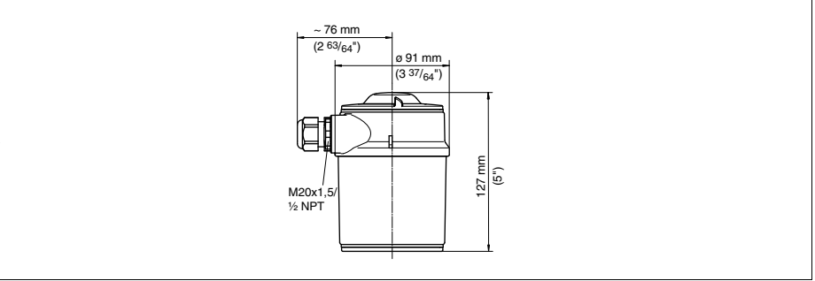
Fig. 35: Boîtier
