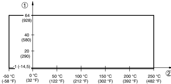
Abb. 30: Prozesstemperatur - Prozessdruck bei Schalterstellung 0,7 g/cm 3 (Empfindlichkeitsumschalter)
