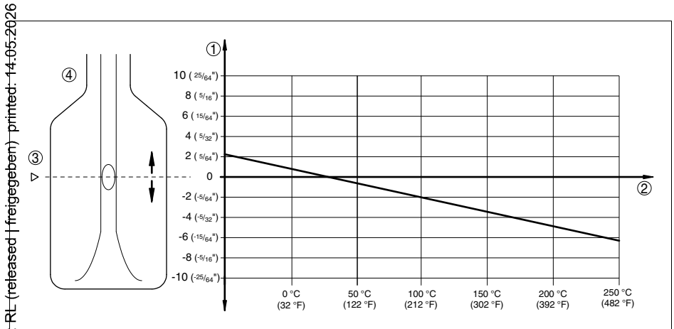
Abb. 26: Einfluss der Prozesstemperatur auf den Schaltpunkt
