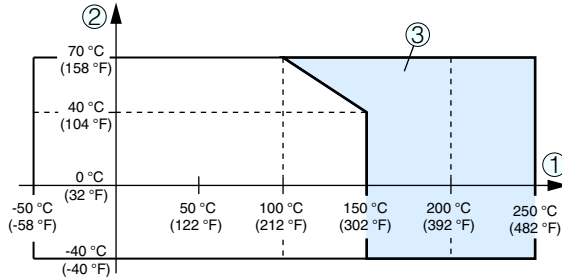
Abb. 29: Umgebungstemperatur - Prozesstemperatur
