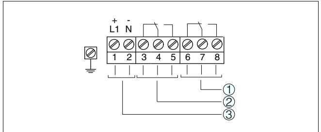
Abb. 11: Anschlussplan Einkammergehäuse
