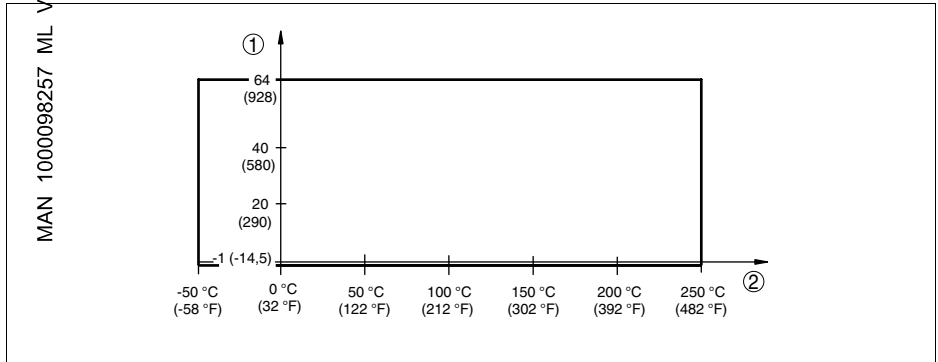
Fig. 33: Température process - pression process avec position du commutateur 0,7 g/cm 3 (commutateur d'inversion de la sensibilité)
