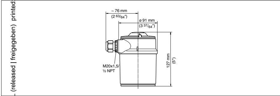
Abb. 32: Gehäuse
