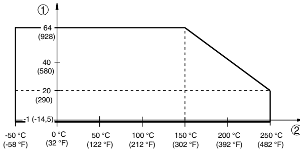
Fig. 34: Température process - pression process avec position du commutateur 0,5 g/cm 3 (commutateur inversion de la sensibilité)
