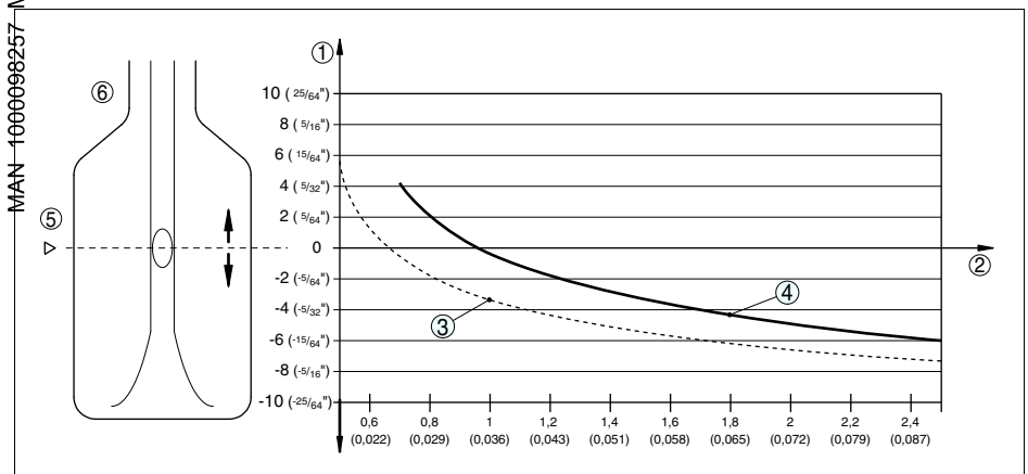
Abb. 27: Einfluss der Füllgutedichte auf den Schaltpunkt
