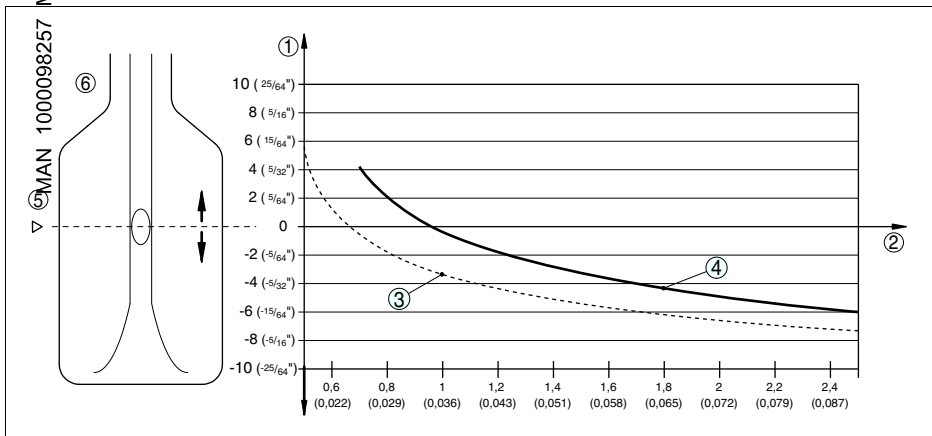
Fig. 30: Influence de la densité du produit sur le point de commutation
