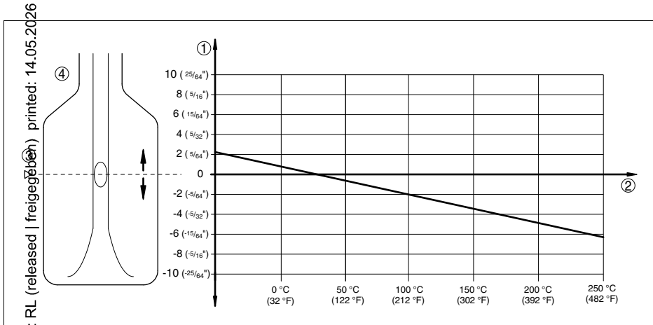
Fig. 29: Influence de la température process sur le point de commutation
