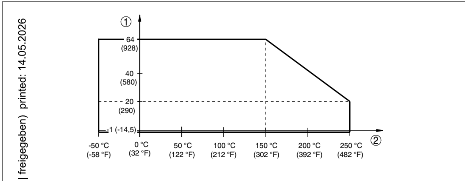
Abb. 811: Prozesstemperatur - Prozessdruck bei Schalterstellung 0,5 g/cm 3 (Empfindlichkeitsumschalter)
