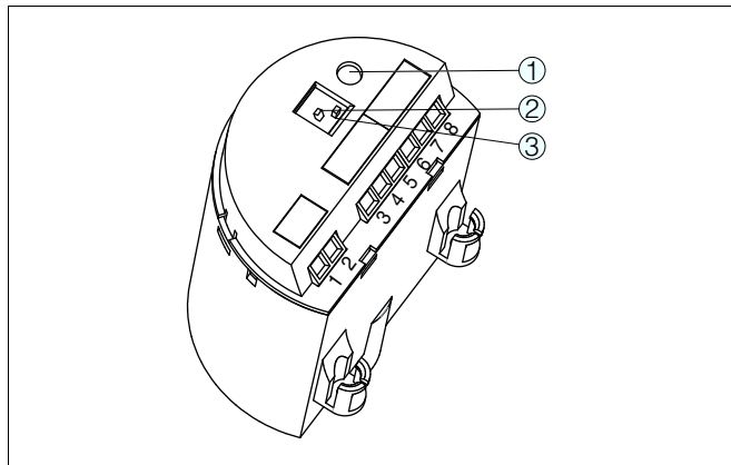
Abb. 12: Elektronikeinsatz SWE60R - Relaisausgang
