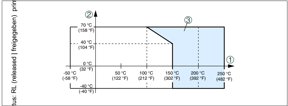
Fig. 32: Température ambiante - température process
