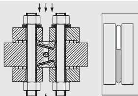
Sichtrichtung Refraktionstyp mit Glimmerscheiben
