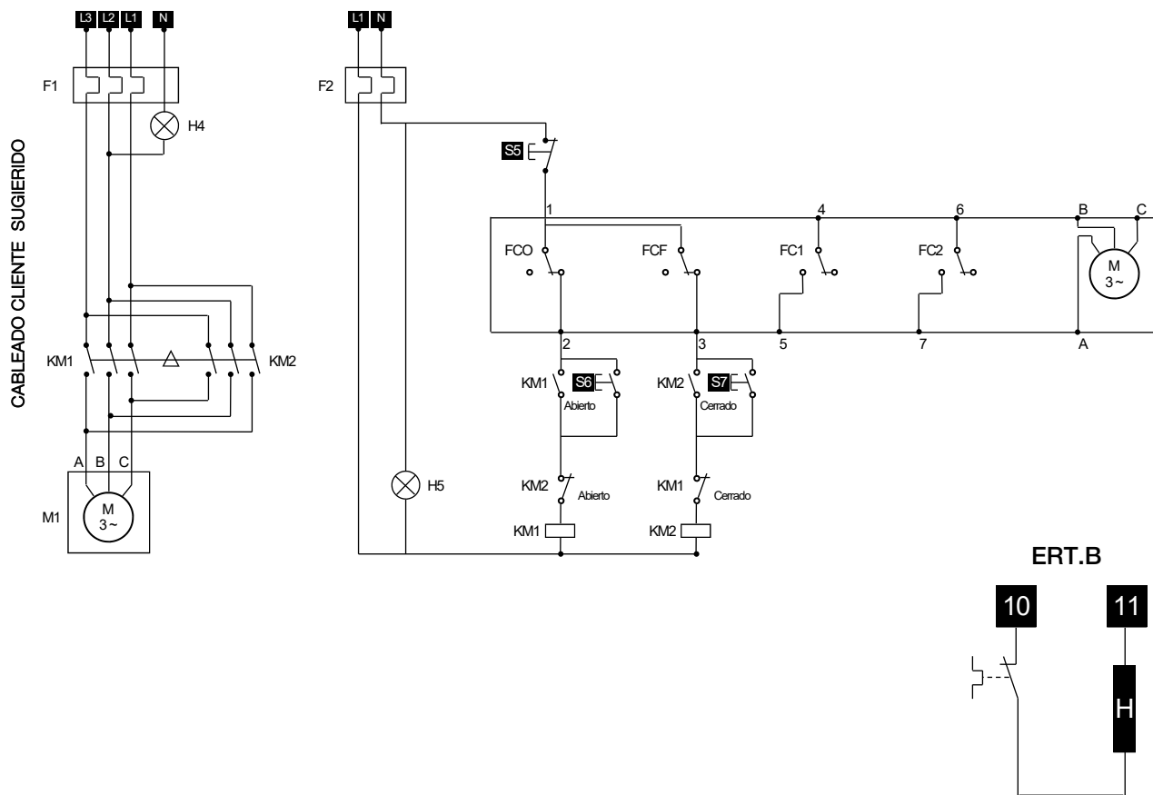
ALIMENTACIÓN (400 V trifásico 50/60 Hz)
